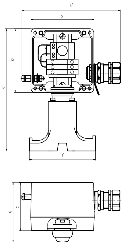
Рисунок 1. Серия PTB 401-ИС
