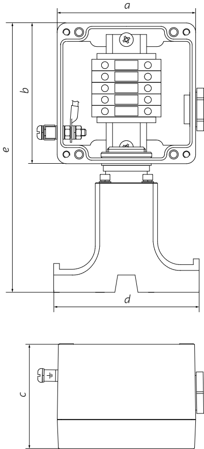
Рисунок 1. Серия ВЭ 122.У
