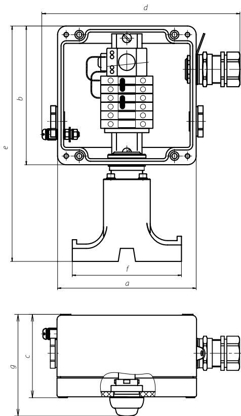
Рисунок 2. Серия PTB 601-ИС
