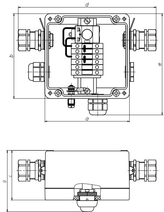
Рисунок 2. Серия PTB 602-ИС
