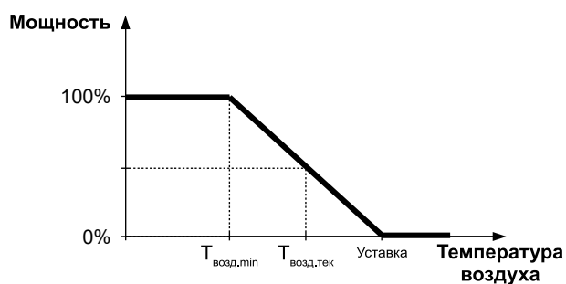
Алгоритм «Воздух»
