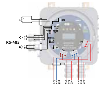
Схема подключения одиночного термостата в сети RS-485
