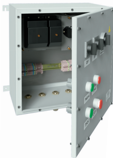
Шкаф SCPE-565 в корпусе из окрашенной конструкционной стали
